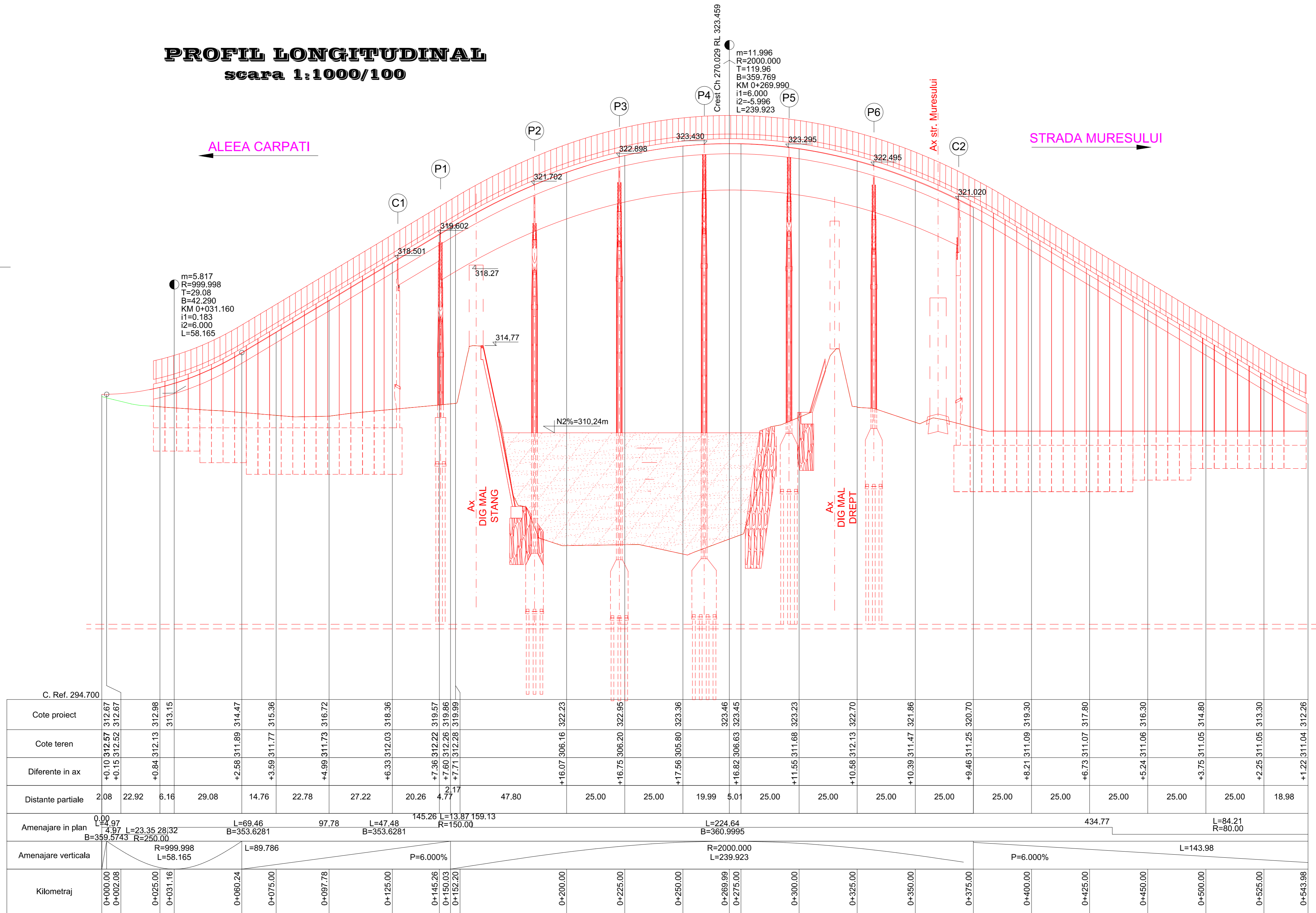
POD MURES Km 0.000 - 375.000 Scara: 1:1000/100
