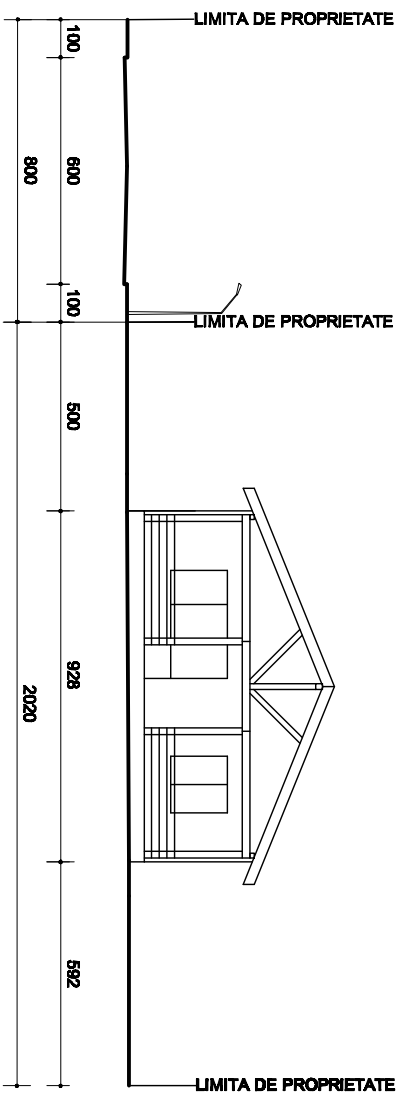
SECTIUNE TRANSVERSALA sc. 1:100
