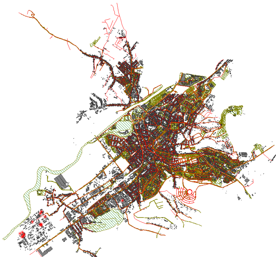
Figura 3. Vedere 2D a modelului de calcul pentru Municipiul Târgu Mureș
