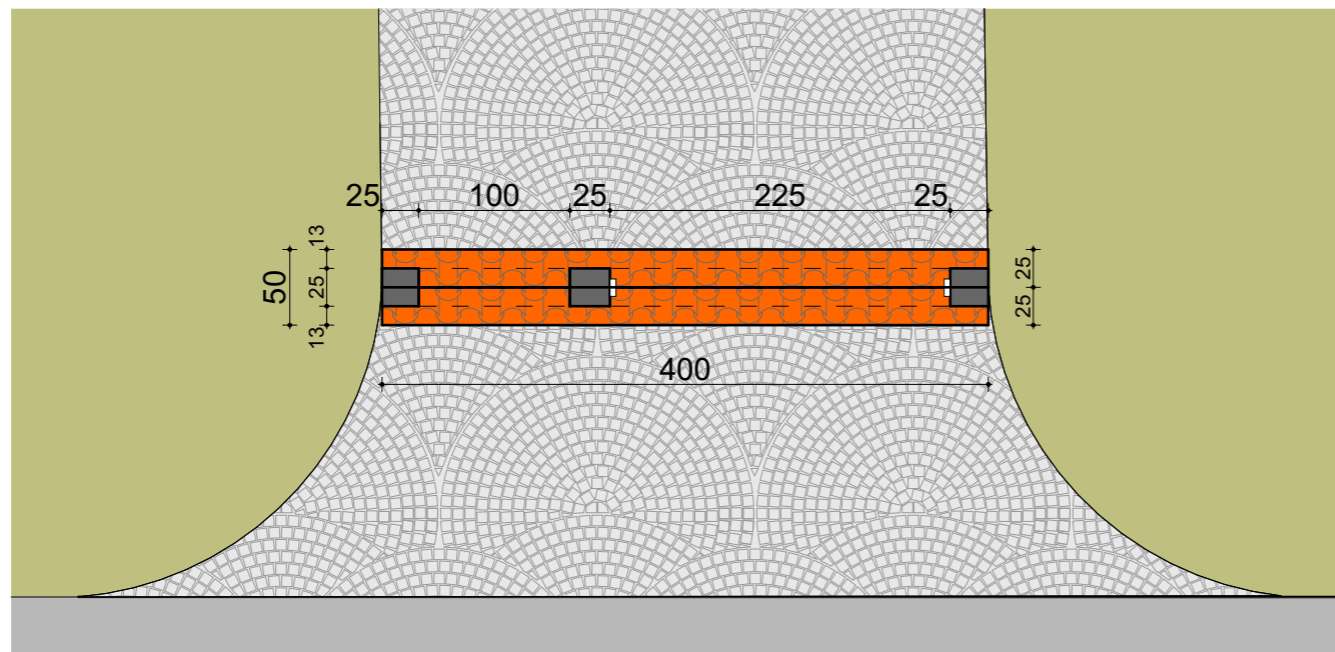
PLAN POARTA
