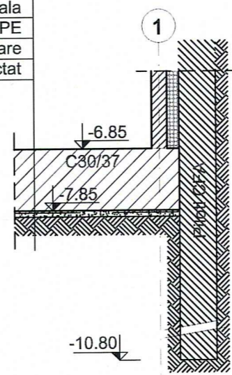
Detaliu fundatie
