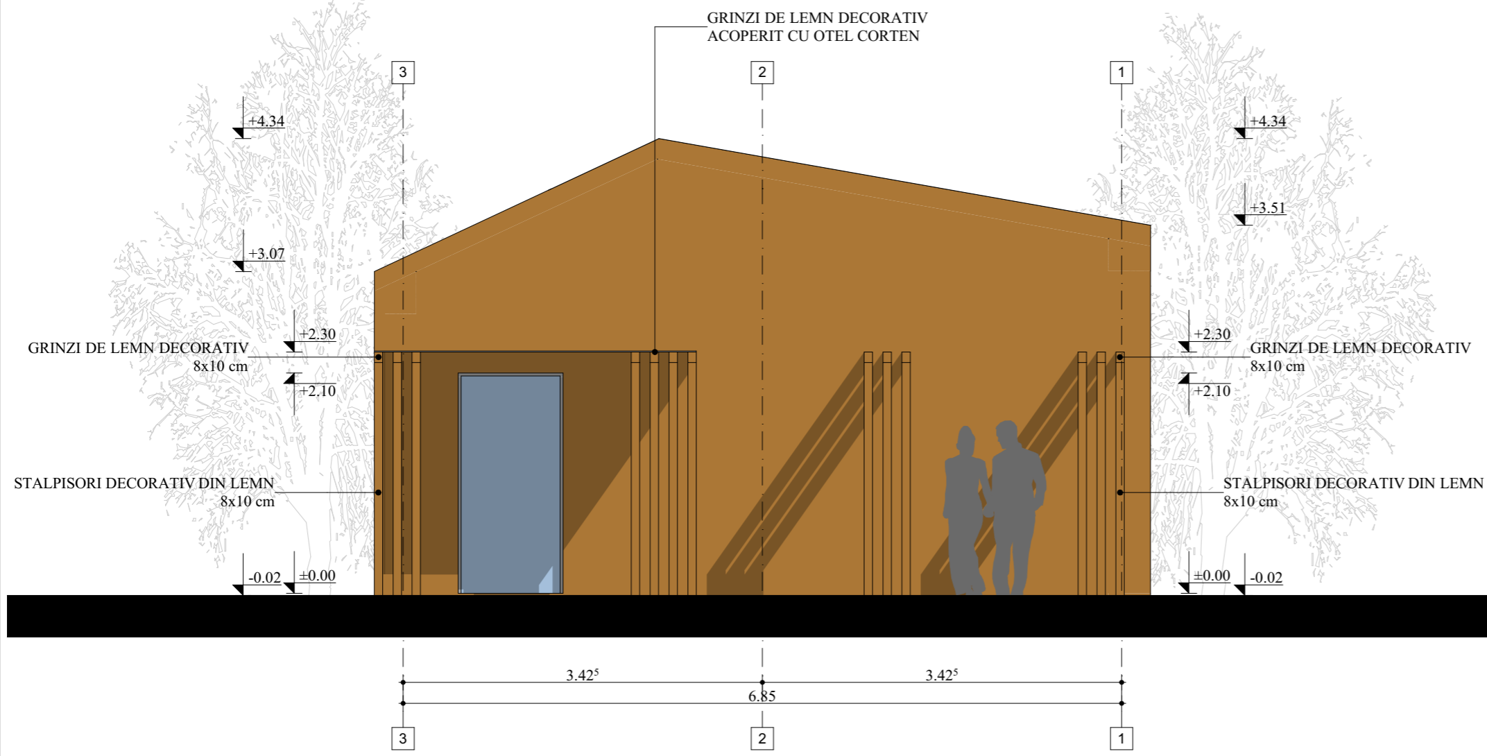
FATADA POSTERIOARA
