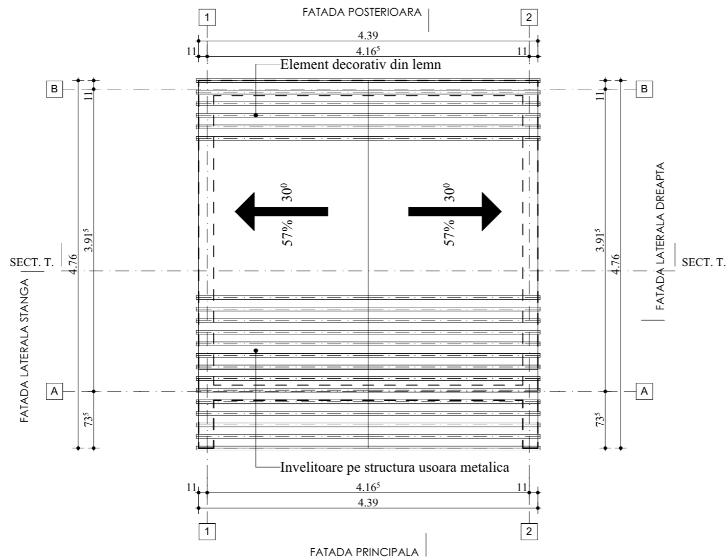
PLAN INVELITOARE
