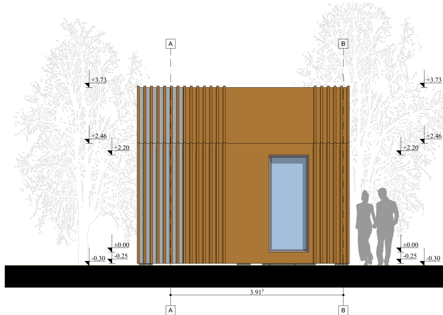
FATADA LATERALA DREAPTA
