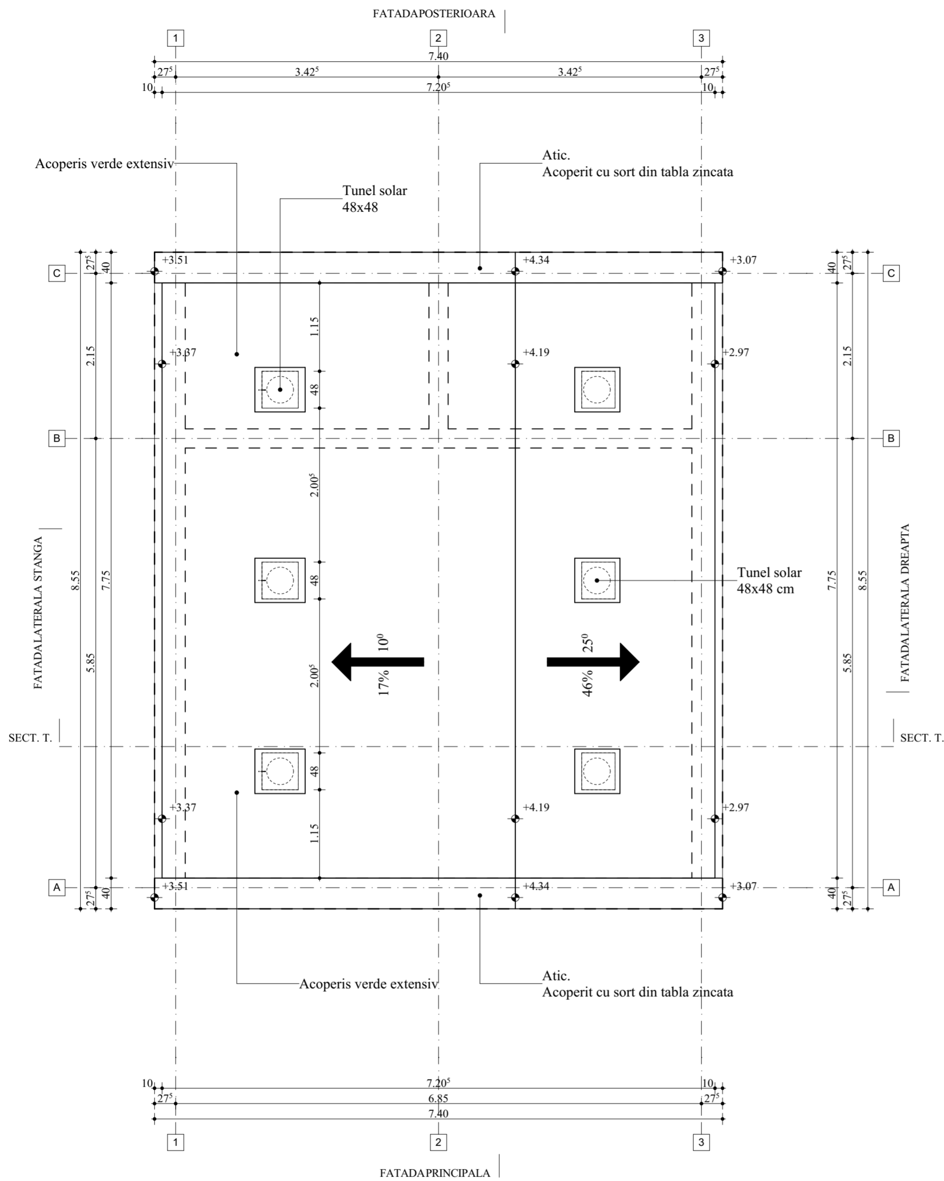
PLAN INVELITOARE
