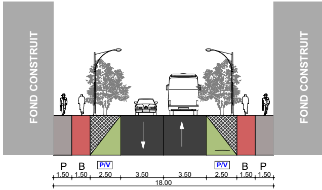
PROFIL SPECIFIC ZONA REZIDENTIALA/MIXTA
