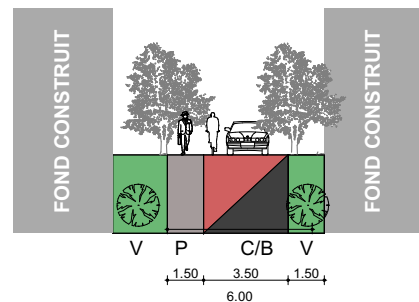
PROFIL SPECIFIC ZONA REZIDENTIALA alee fundatura <35m
