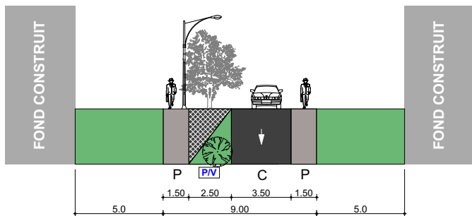
PROFIL SPECIFIC ZONA REZIDENTIALA fundatura <35m sau bucla cu sens unic
