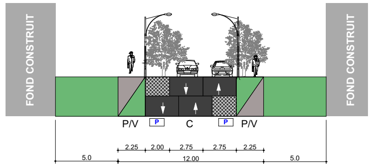
PROFIL SPECIFIC ZONA LOCUINTE INDIVIDUALE
