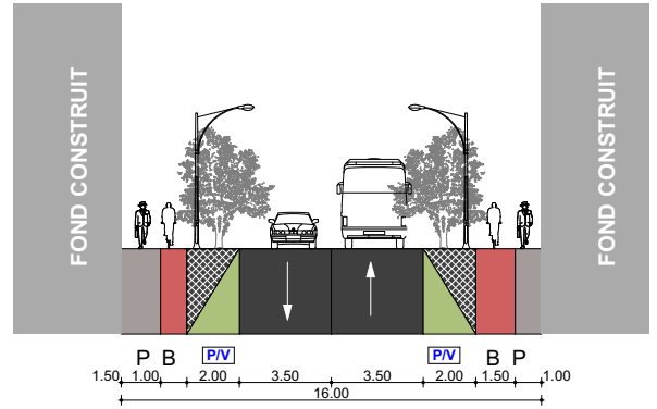
PROFIL SPECIFIC ZONA REZIDENTIALA -COLECTOARE
