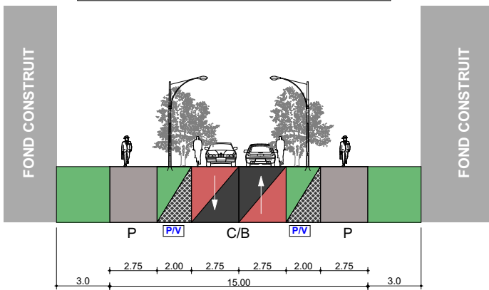
PROFIL SPECIFIC ZONA LOCUINTE COLECTIVE
