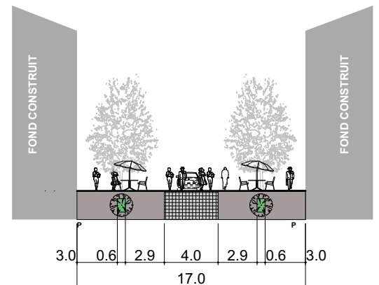
STRADA ENESCU -situatia propusa profil transversal acordare prioritate circulatiei pietonale (CONCURS ARHITECTURA)
