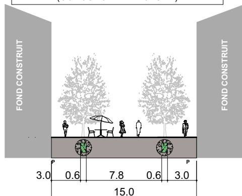
STRADA BOLYAI FARCAS -situatia propusa circulatie exclusiv pietonala /alternativa (CONCURS ARHITECTURA)
