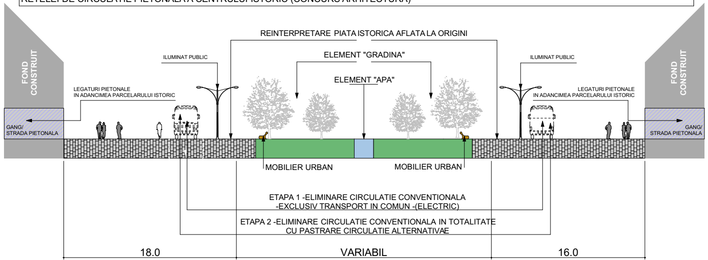
ZONA CENTRALA - STRADA TUDOR VLADIMIRESCU - situatia propusa etapa 1
