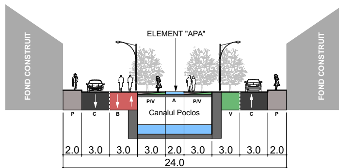
ZONA CENTRALA - STRADA TUDOR VLADIMIRESCU - situatia propusa etapa 2
