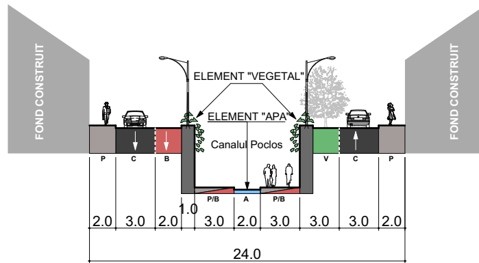
ZONA CENTRALA - STRADA TUDOR VLADIMIRESCU - situatia propusa etapa 1
