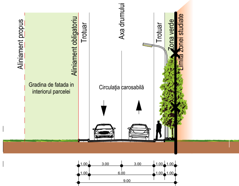
Profil strada Sectiune A - A Scara 1:200
