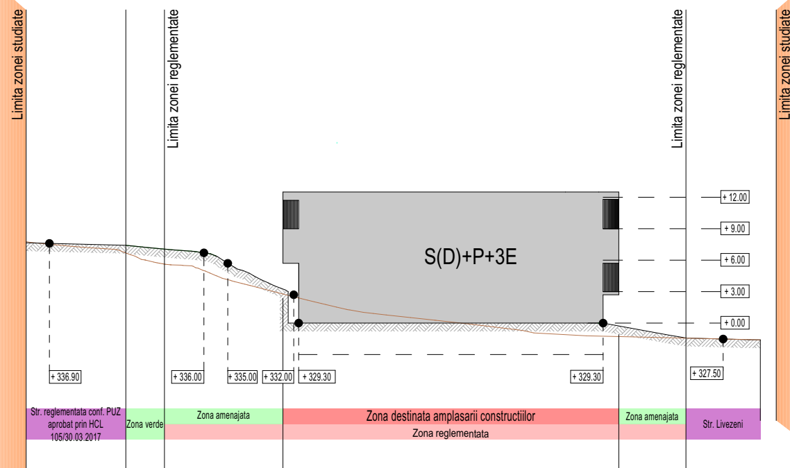
SECTIUNE PRIN TEREN - PROPUȘ 1 - 1
