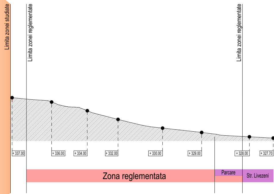
SECTIUNE PRIN TEREN - EXISTENT 1' - 1'
