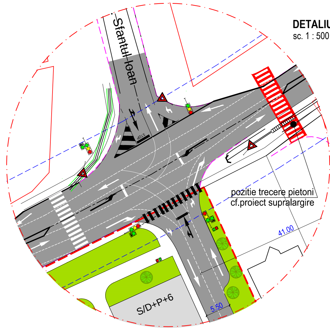
POSSIBILITATE DE AMENAJARE INTERSECTIE SEMAFORIZATA
