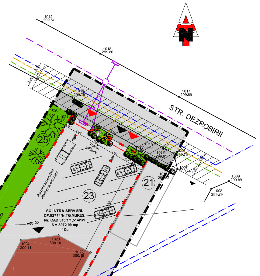
PLAN DE SITUATIE Sc 1:500
