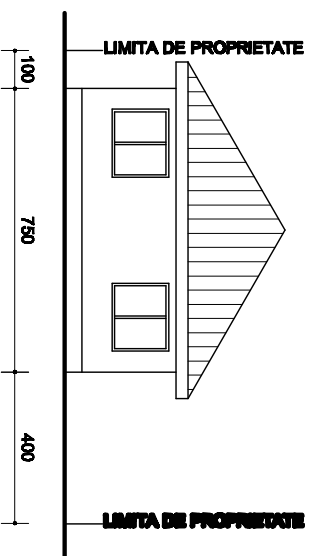
SECTIUNE TRANSVERSALA sc. 1: 100
