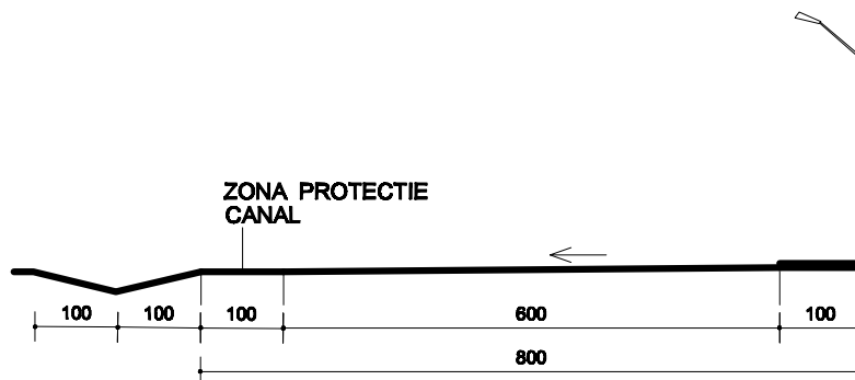
STRADA LOCALA PROFIL TRANSVERSAL PROPUS SC. 1 : 100
