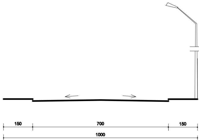
STRADA PROPUSA IN PUZ UNIRII PROFIL TRANSVERSAL PROPUS SC. 1 : 100
