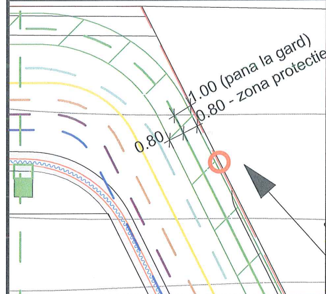
Detaliu les. Scara: 1:200
