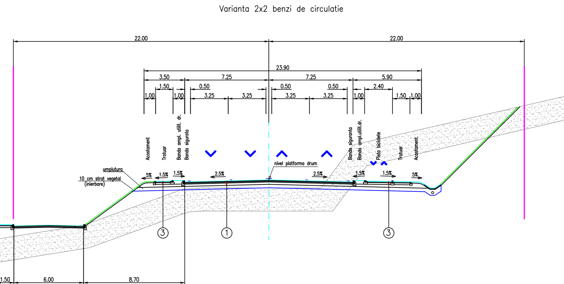
SECTIUNE TRANSVERSALA CORELARE CU PROPUNEREA DE LARGIRE LA 4 BENZI A CAII SIGHISOAREI
