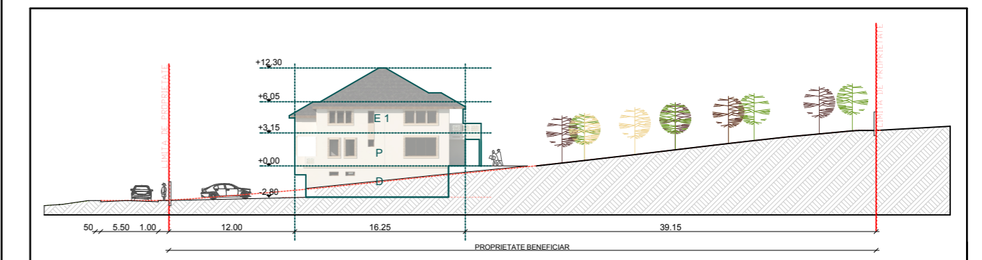
SECTIUNE A-A 1: 500
