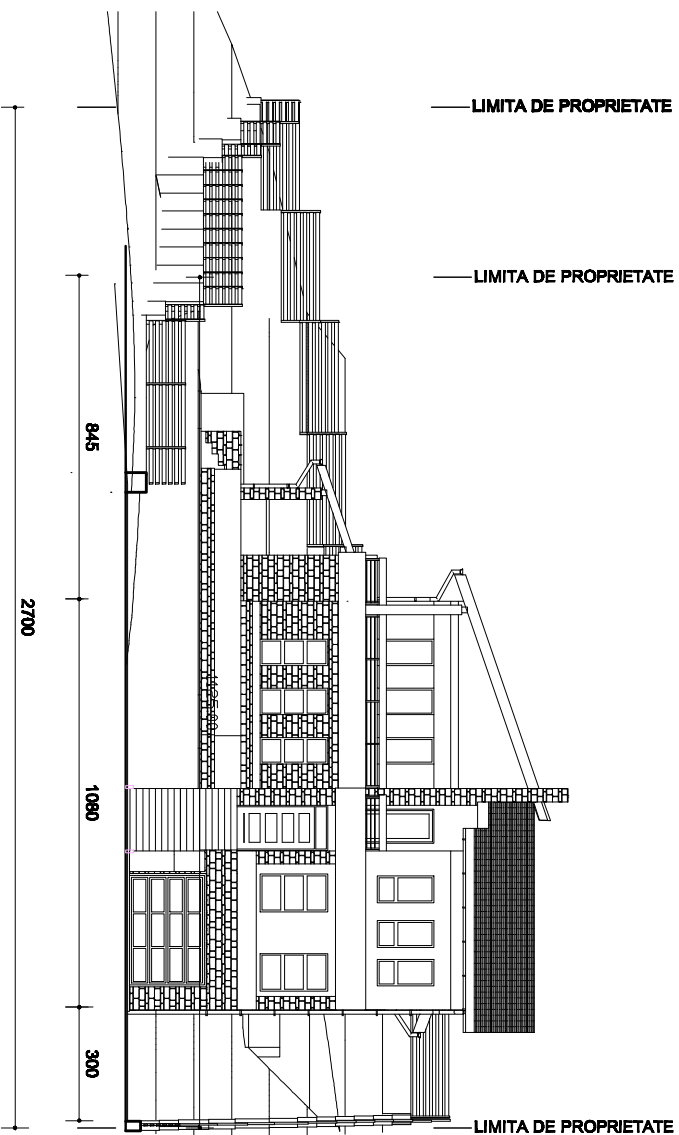
VEDERE - SECTIUNE FRONTALA sc. 1 : 200
