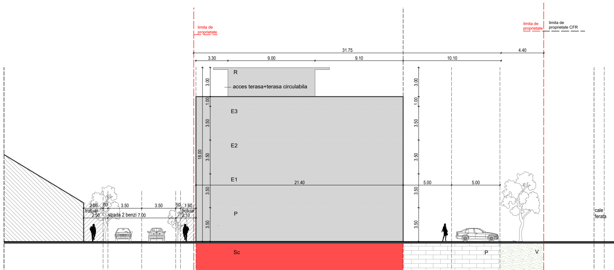
PROFIL TRANSVERSAL
