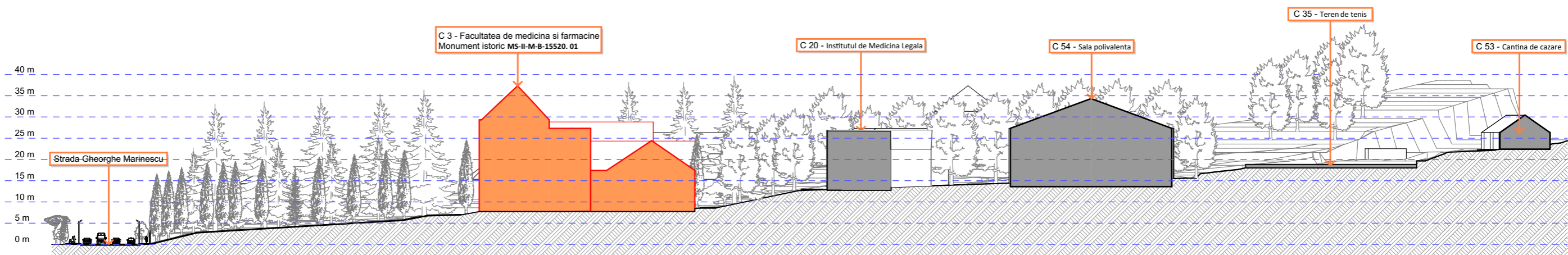
SECTIUNE 1-1' SC 1:1000
