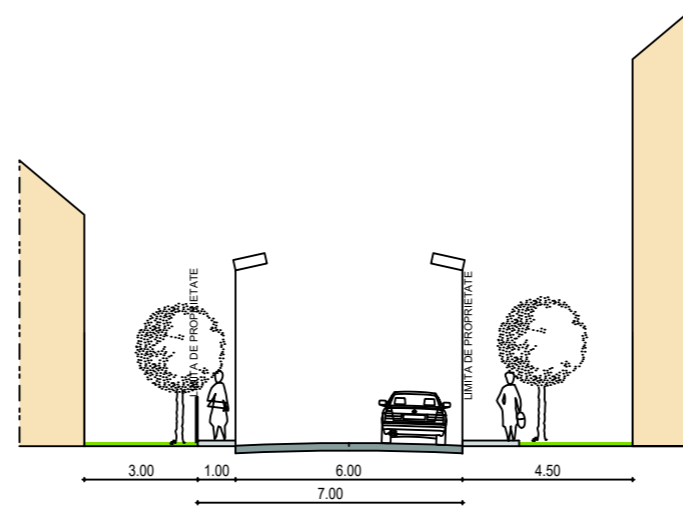
PROFIL STRADAL2
