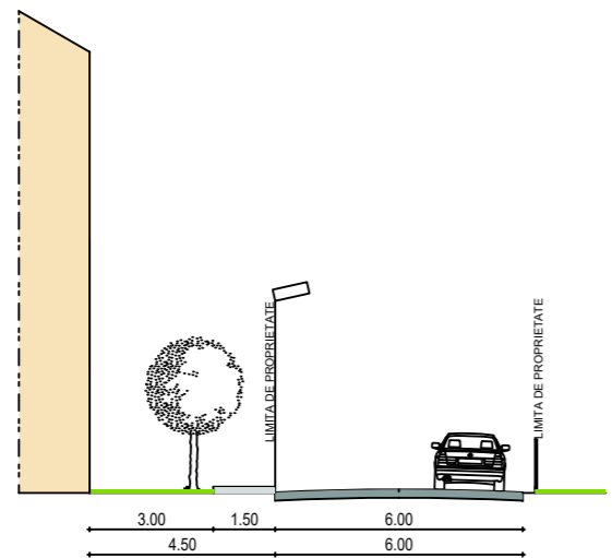
PROFIL STRADAL4
