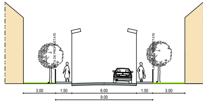
PROFIL STRADAL1
