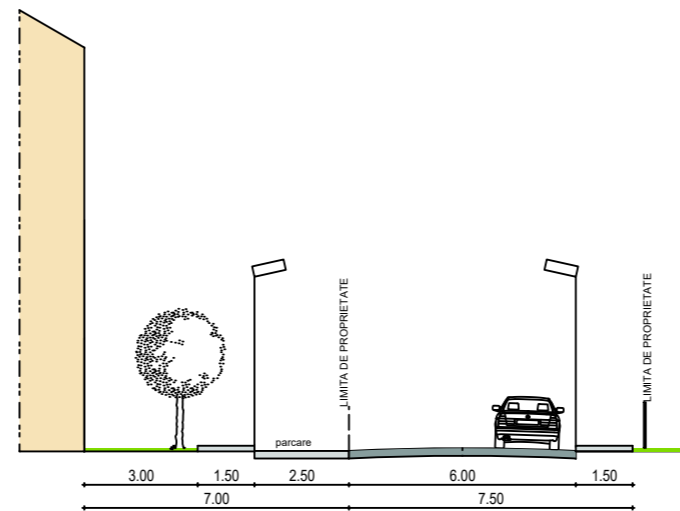
PROFIL STRADAL5
