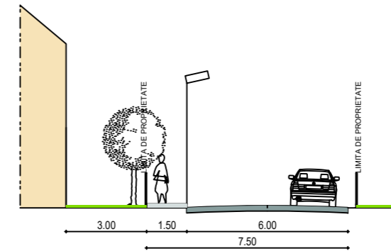
PROFIL STRADAL3
