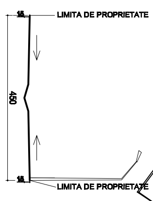
STRADA DE ACCES LA LOT PROFIL TRANSVERSAL PROPOS SC. 1 : 100
